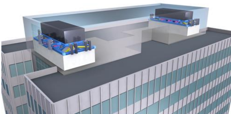
【「デュアル TMD-NT」屋上設置イメージ】
